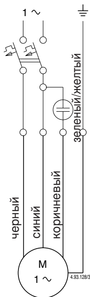
Схема подключения насосов серии SDM с монофазными двигателями
